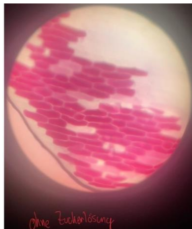
Abb. 5: Schülerversuch: Plasmolyse und Deplasmolyse von Zellen der roten Küchenzwiebel (Fotos: Wenedikt Eichmann)
