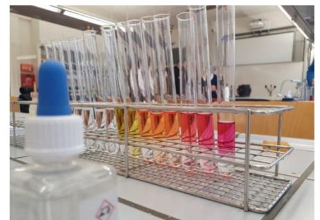
Abb. 4: Schüler:innen erstellen eine pH-Skala mit Universalindikatorlösung (Foto: Dorothe Radelof)
